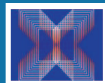
Codex
