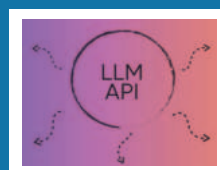
LLM API
